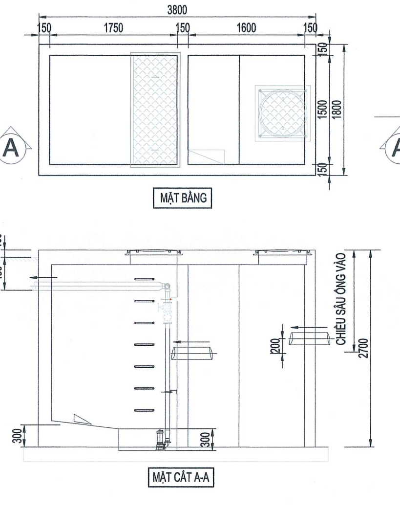
CHI TIẾT HỒ BƠM NƯỚC THẢI 2 TL:1/50 (BON VỊ MM)
