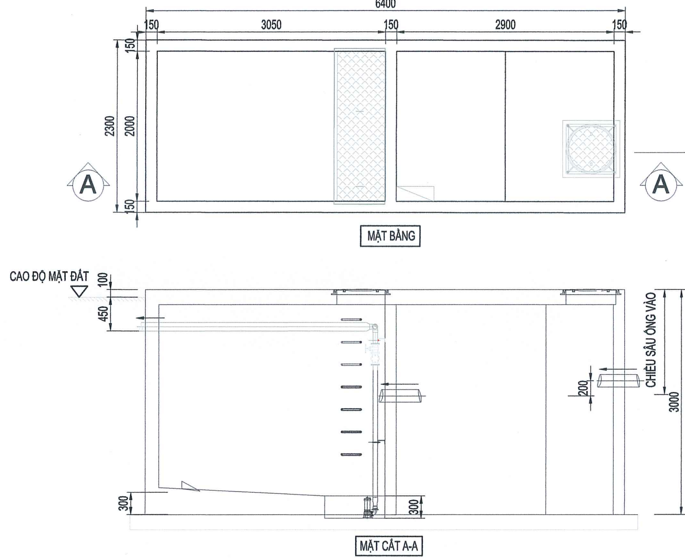
CHI TIẾT HỒ BƠM NƯỚC THẢI 1 TL:1/50 (BON VỊ MM)
